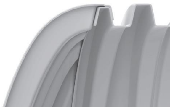
Figura 2. Colocación de las tapas
