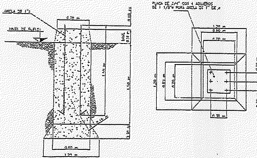
DETALLE DE BASE DE CONCRETO
