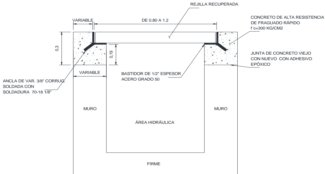
REJILLA PARA DRENAJE PLUVIAL
