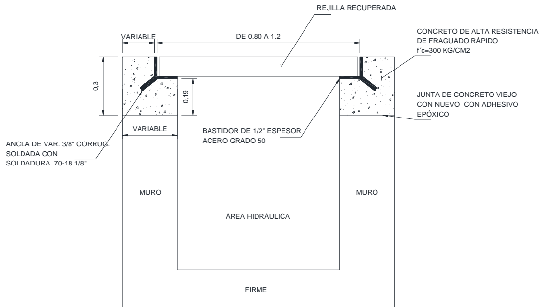
REJILLA PARA DRENAJE PLUVIAL
