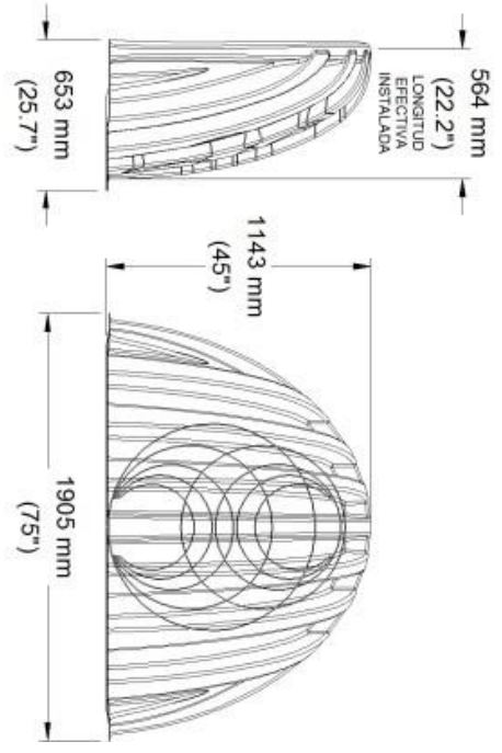
Figura 4. Dimensiones de la tapa MC-3500.
