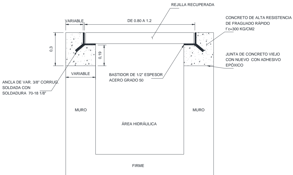
REJILLA PARA DRENAJE PLUVIAL
